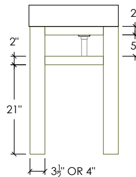
RIGHT ELEVATION
