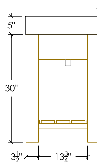
RIGHT ELEVATION
